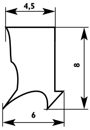
Ущільнювач для скла в паз 8 мм
