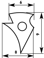
Ущільнювач для скла в паз 10 мм
